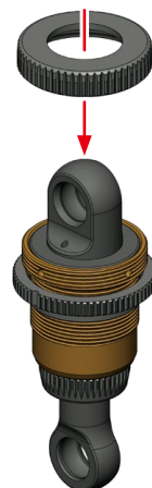
T319 USP2 Shock Cap USP2 ショックキャップ
