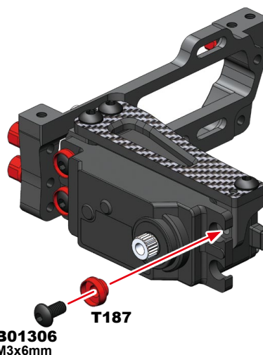
T278 Alu Servo Mount Block アルミサーボマウントブロック
