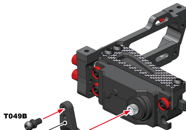
T007 Servo Horn, Steering Arm Set サーボホーン, ステアリングアームセット
